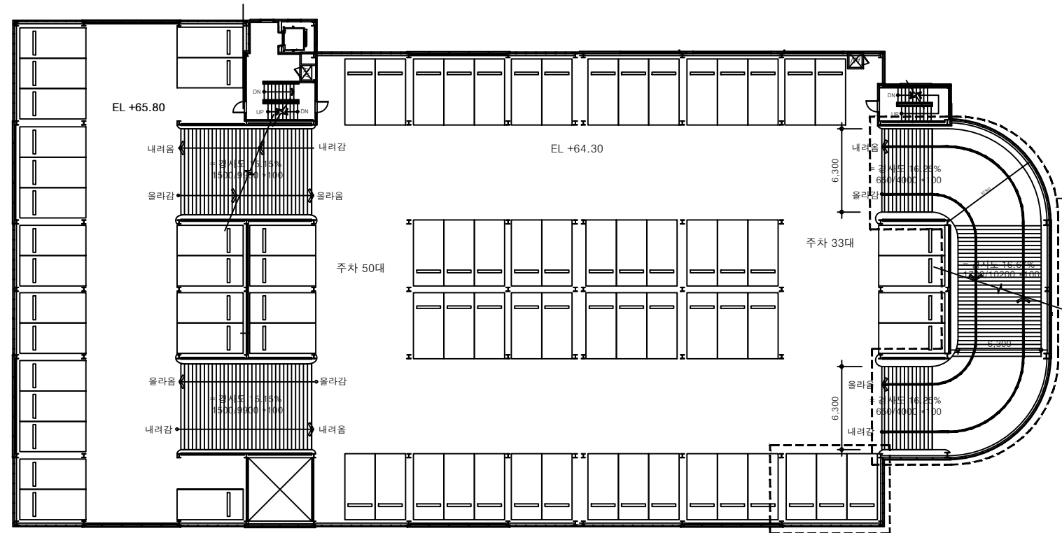
3층 평면도(기존) SCALE A1 : 1/200 A3 : 1/400
