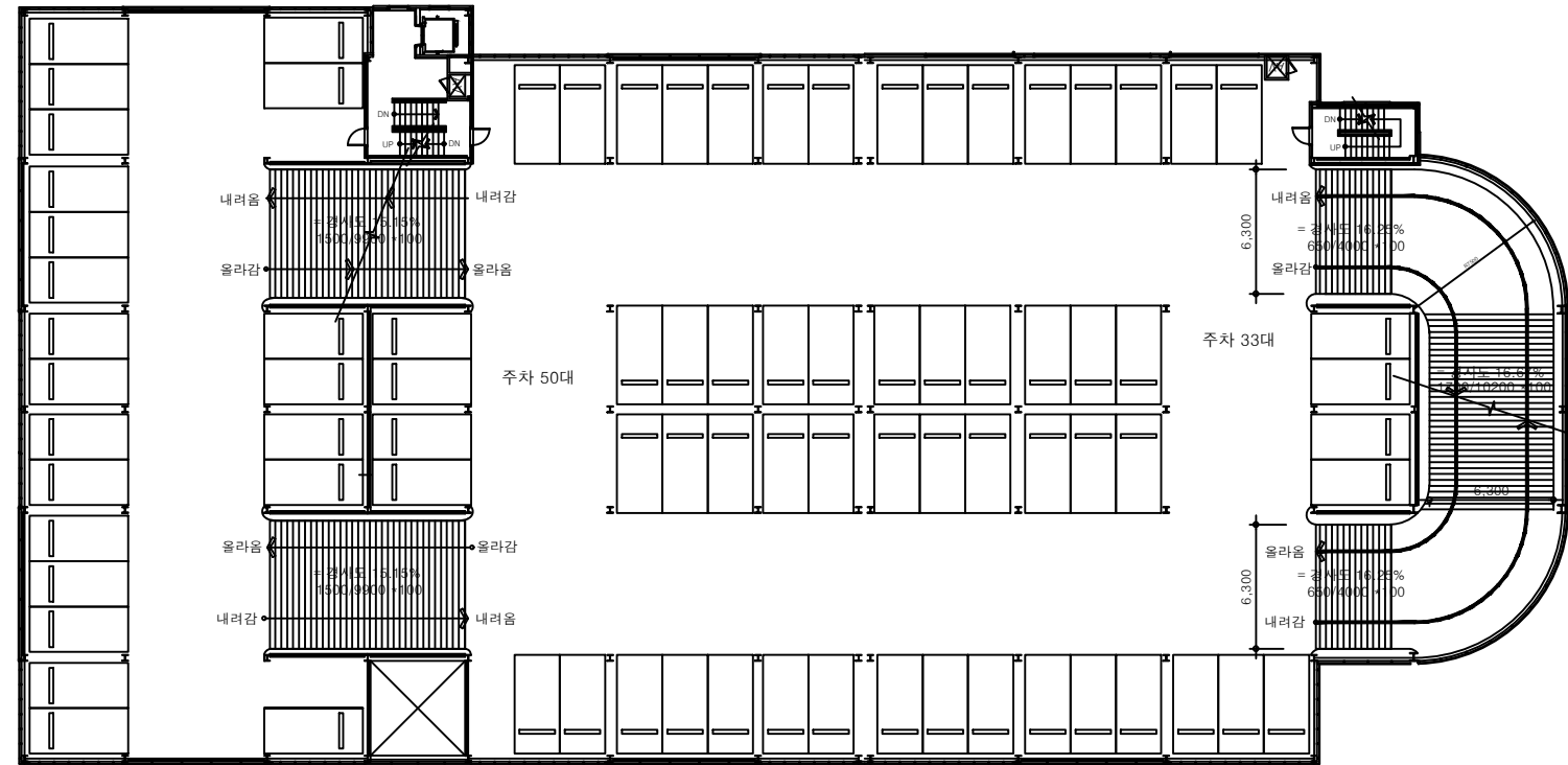
5층 평면도 SCALE A1 : 1/200 A3 : 1/400
