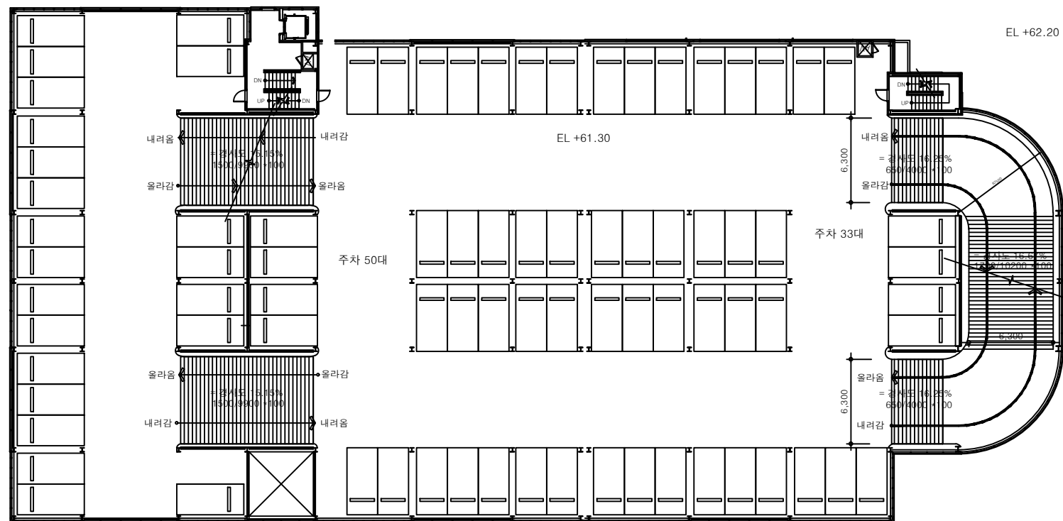
2층 평면도(기준) SCALE A1 : 1/200 A3 : 1/400
