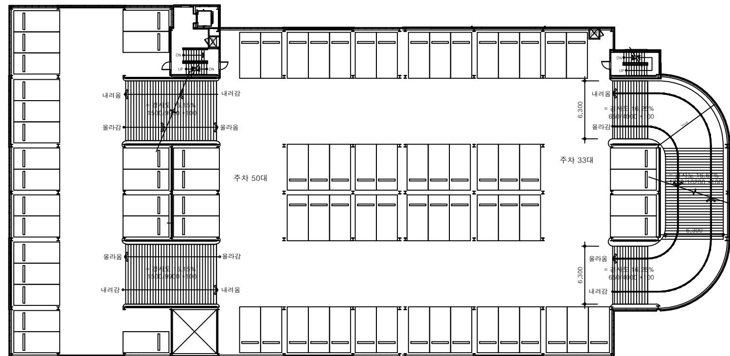
6층 평면도(신설) SCALE A1 : 1/200 A3 : 1/400
